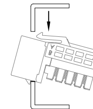
資訊插座安裝步驟
