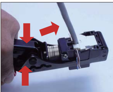
4. 握緊把手壓線 & 切線
