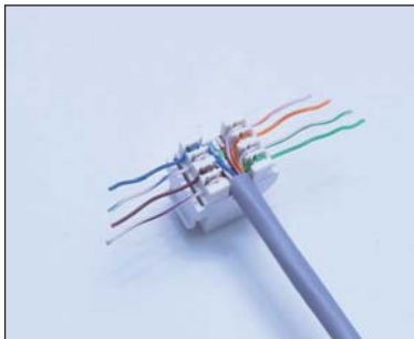
2. 分線於端子上
