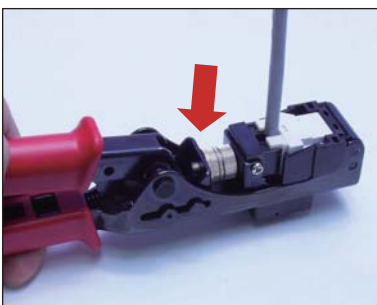
刀片深度調整鈕
