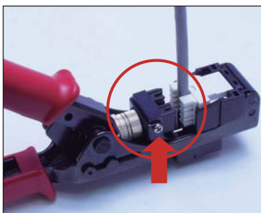
可鬆開螺絲更換刀頭
